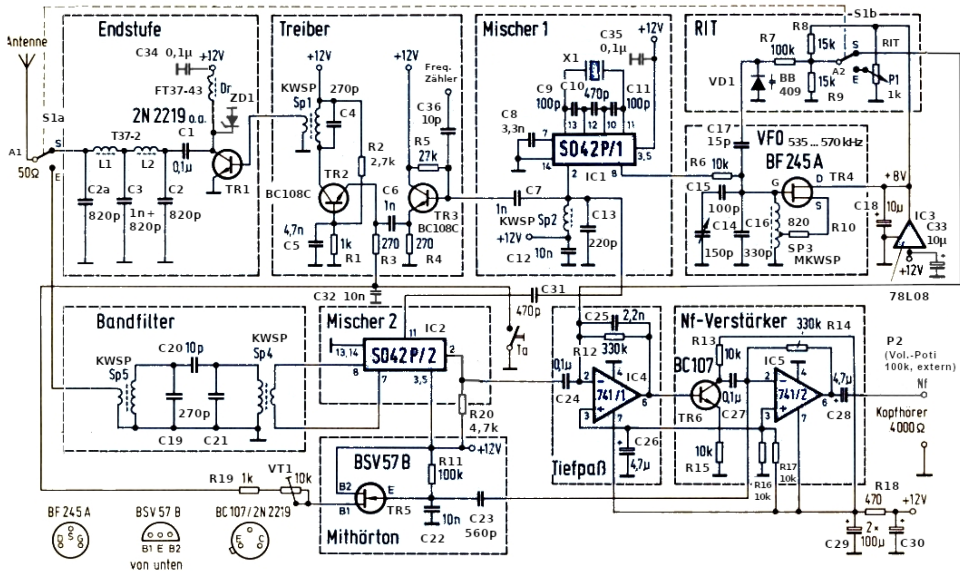
Bild 2. Vollständiges Schaltbild des Transceivers für das 80-m-CW-Band
